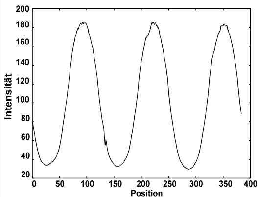
Nahezu sinusförmige Helligkeitsmodulation der LCD-Linien mit Option SINUS
